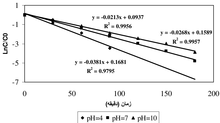
شکل ۴: تأثیر pH بر میزان حذف رنگ راکتیو قرمز ۱۹۸ در فرایند TiO_2/UV-C ( C_0=100 \text{ mg/L} , TiO_2=0.4 \text{ g/L} )
