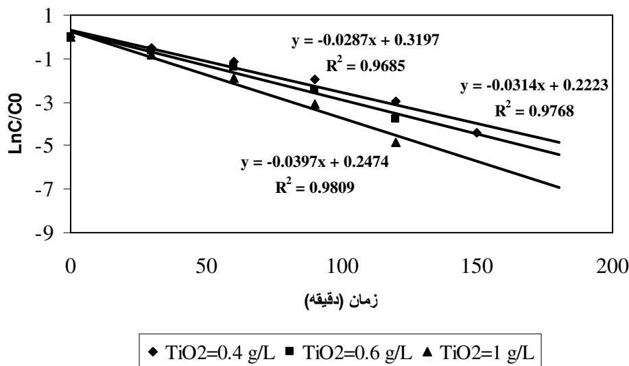
شکل ۵: تأثیر مقدار TiO 2 بر میزان حذف رنگ راکتیو قرمز ۱۹۸ در فرایند TiO 2 /UV-C (C 0 =۱۵۰ mg/L, pH: ۴)
