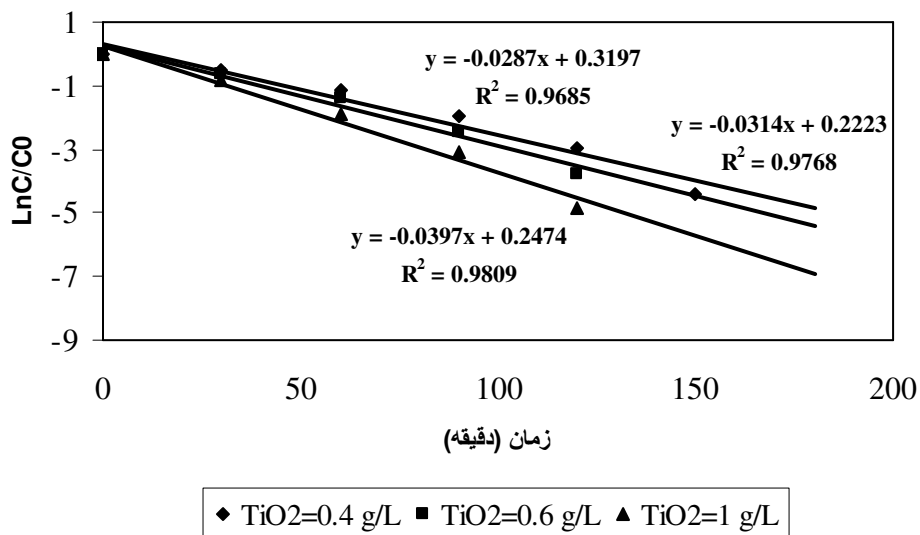
شکل ۵: تأثیر مقدار TiO 2 بر میزان حذف رنگ راکتور فرمز ۱۹۸ در فرایند TiO 2 /UV-C (C 0 =۱۵۰ mg/L, pH: ۴)
